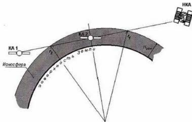
Рис. 3. Прохождение сигнала НКА — КА через ионосферу
