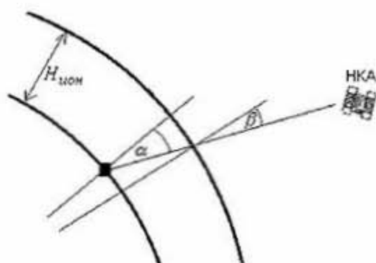
Рис. 1. Прохождение сигнала НКА — приемник через ионосферу
