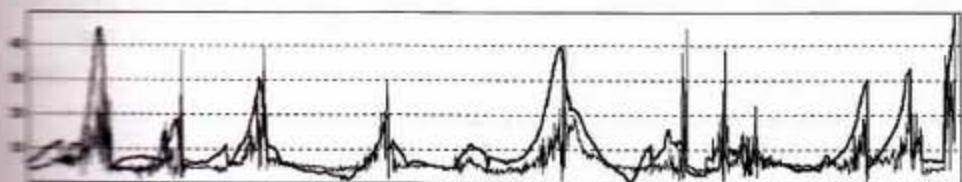
Рис. 5. Ионосферная составляющая ошибки измерения псевдодальности НКА GPS № 31
